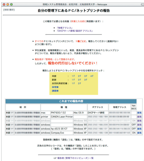
図 3：個人管理ネットワーク機器 / 端末の報告ページ (トップ)
